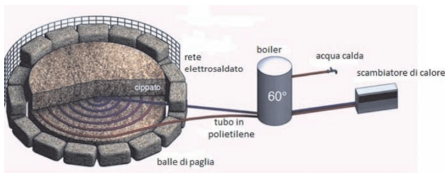
Impianto di termocompostaggio
